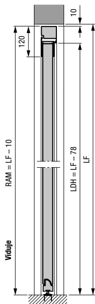
Šoninės durys su aliuminine blokine stakta, 2 profilio tipas Montavimas angoje
