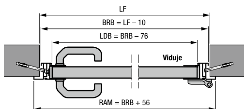
Šoninės durys su aliuminine kampine stakta, 2 profilio tipas Vidinė atrama
