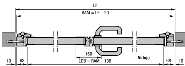
Dviverės šoninės durys su aliuminine blokine stakta, 2 profilio tipas Montavimas angoje
