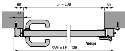
Šoninės durys su aliuminine blokine stakta, 2 profilio tipas Montavimas už angos
