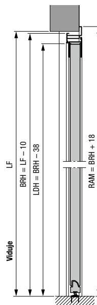
Šoninės durys su aliuminine kampine stakta, 2 profilio tipas Išorinė atrama
