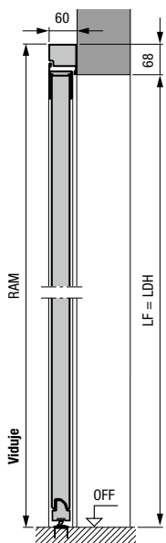
Šoninės durys su aliuminine blokine stakta, 2 profilio tipas Montavimas už angos
