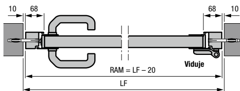
Šoninės durys su aliuminine blokine stakta, 2 profilio tipas Montavimas angoje
